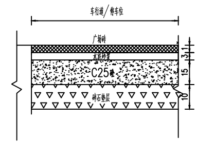
端部大样图三
