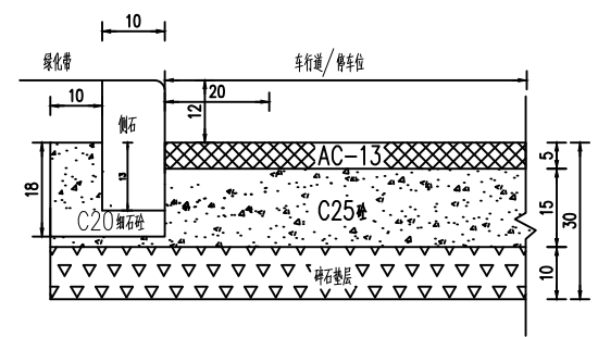
端部大样图一
