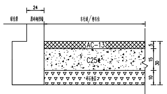
端部大样图二
